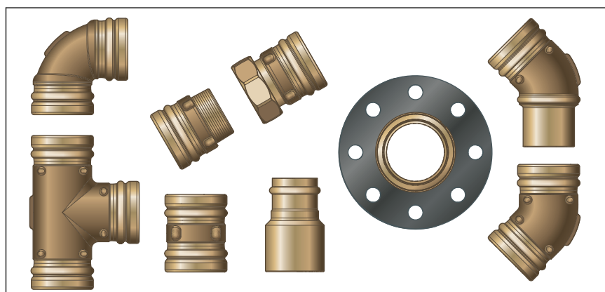
Fig. 1: raccordo a pressare Sanpress XL
