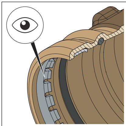
Fig. 5: Anillo cortante
