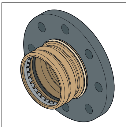
Abb. 6: Losflansch
