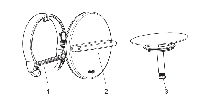
Fig. 1: Panoramica componenti
