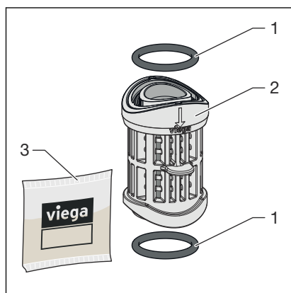
Afb. 1: Buisonderbrekerinzetstuk
