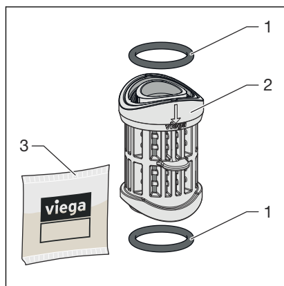
Kuva 1: Putkitulppaosa
