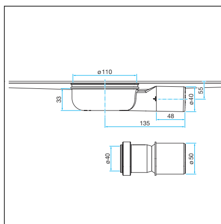
Fig. 1: Dibujo acotado para el modelo 4982.93
