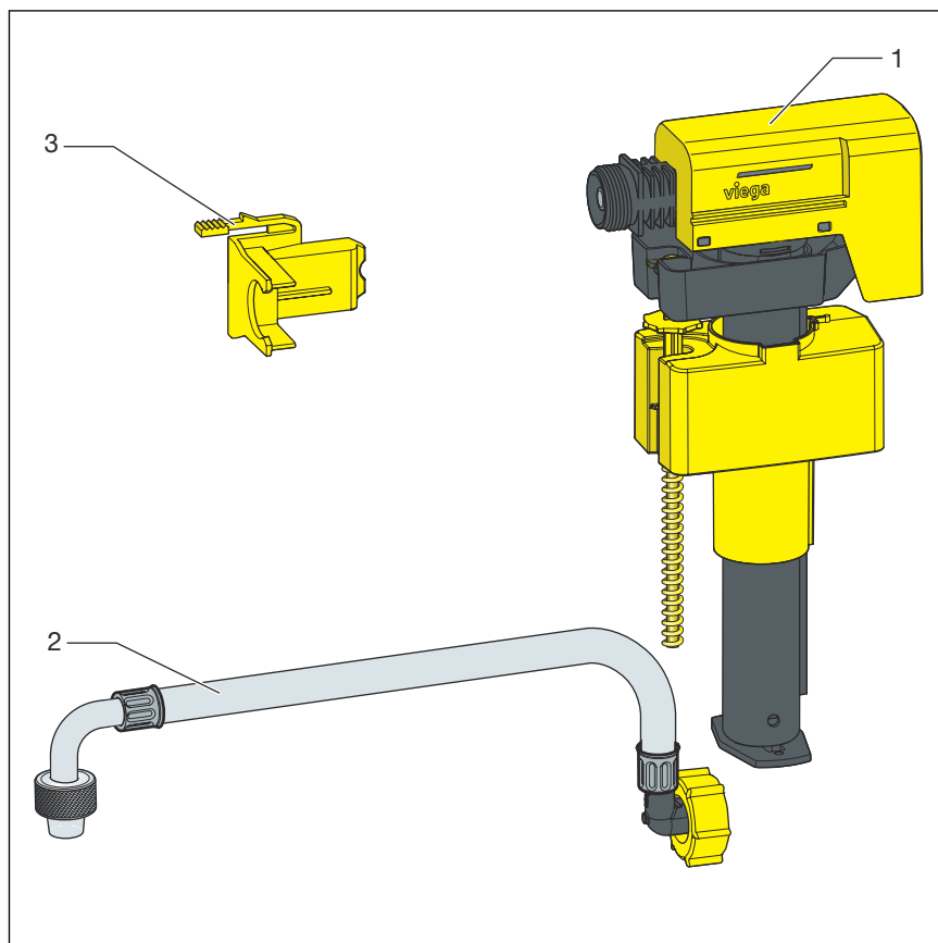
Kuva 1: Täyttöventtiilisarja
