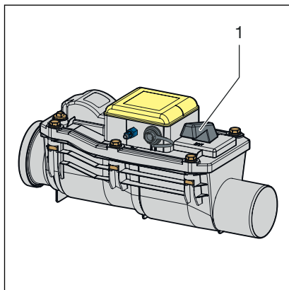
Afb. 5: Bedieningselementen terugloopsluiting
