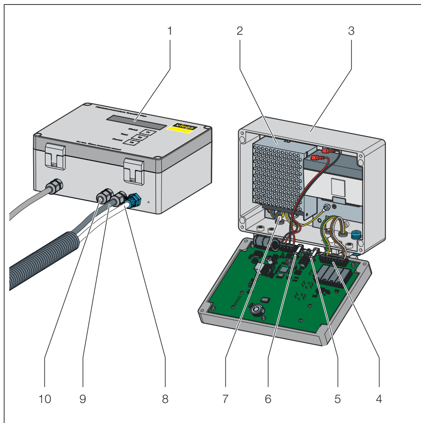
Afb. 4: Componenten regeleenheid
