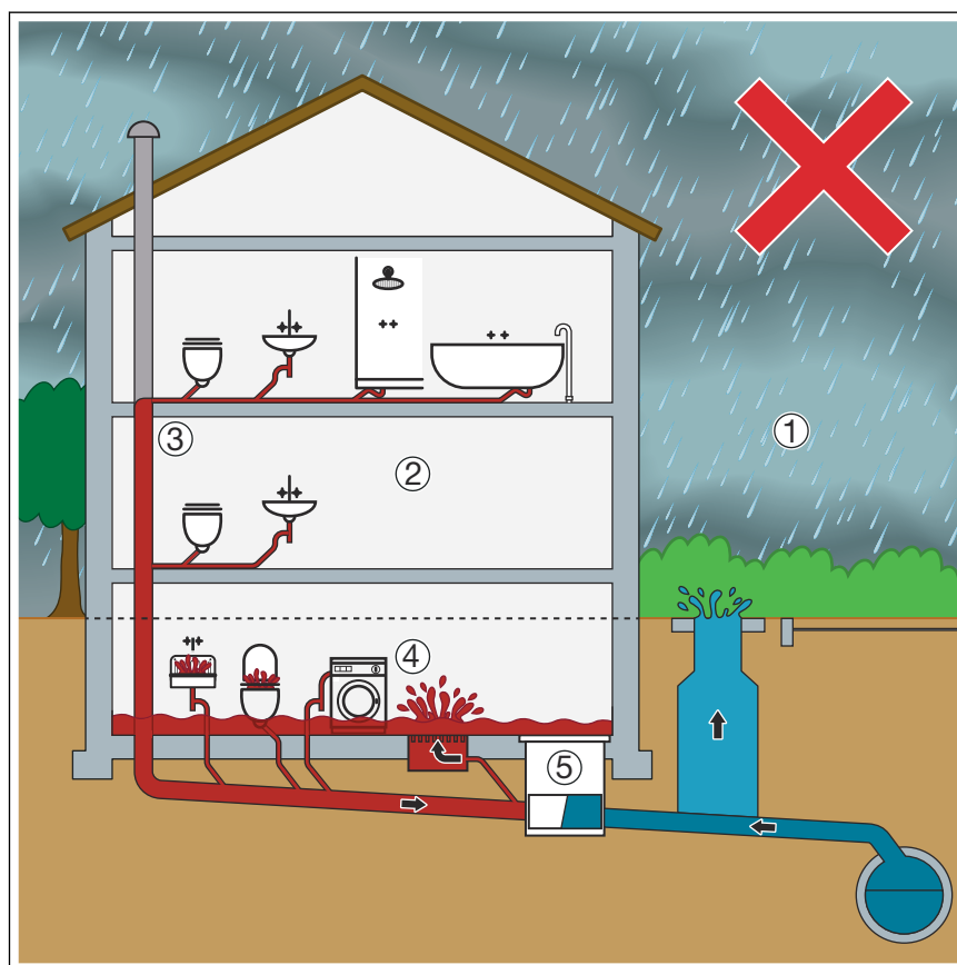
Afb. 1: Verkeerde inbouwplaats van de terugloopsluiting
