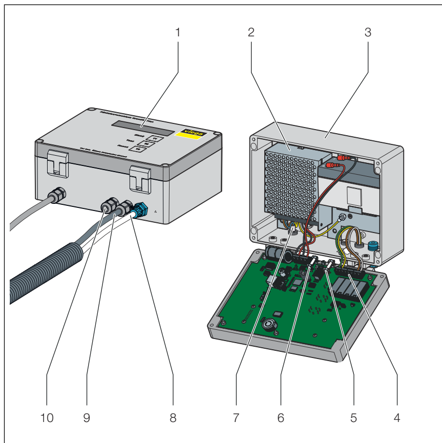
Abb. 4: Bauteile Steuereinheit
