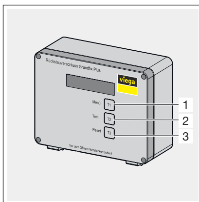
Abb. 6: Bedienelemente Steuereinheit
