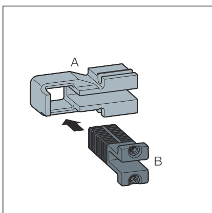
Abb. 24: Stegrosthalter-Paar
