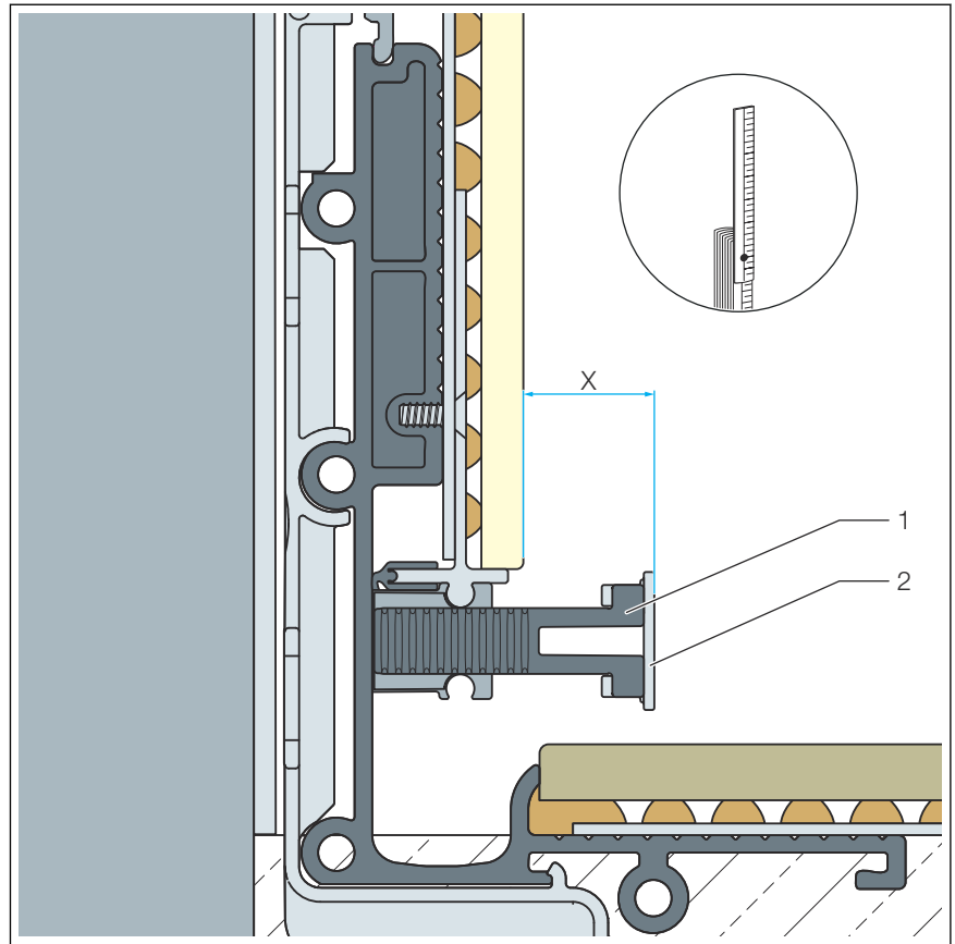
Abb. 26: Maß des Stegrosthalters ermitteln
