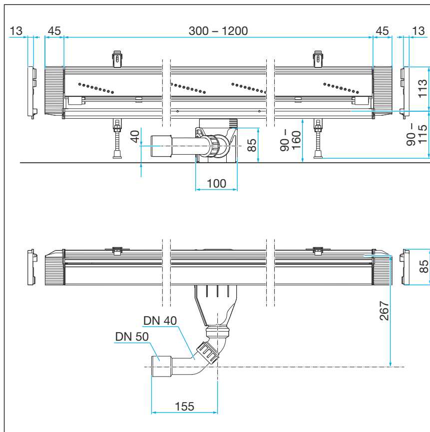
Abb. 18: Abmessungen Grundkörper Basismodell
