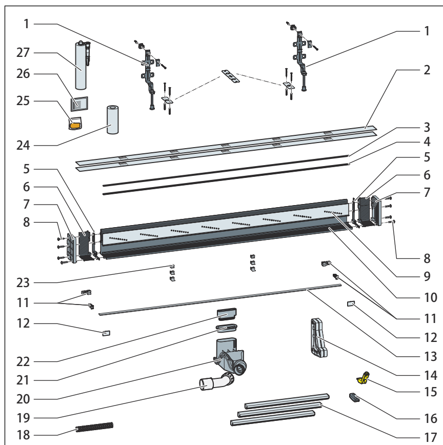
Abb. 13: Bauteile und Lieferumfang
