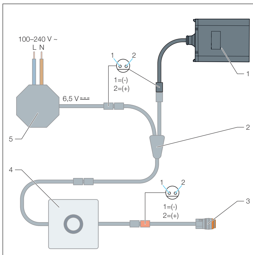
Slika 2: Priključna shema, sjedište baterije, mrežni dio, potisna ploča pisoara za Prevista
