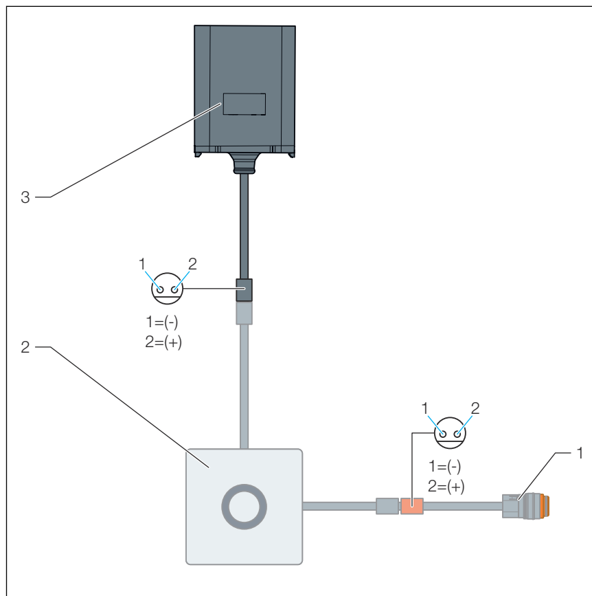
Slika 1: Priključna shema, sjedište baterije, potisna ploča pisoara za Prevista
