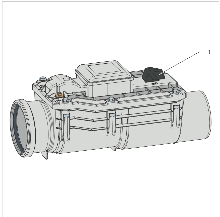
Abb. 4: Bedienelemente Rückstauverschluss
