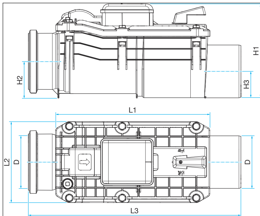
Abb. 5: Einbaumaße
