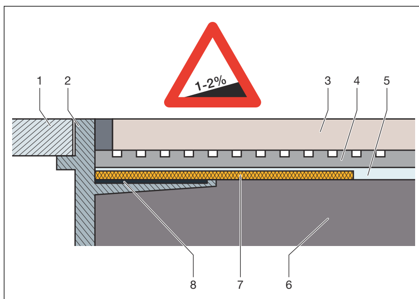
Abb. 2: Aufbauschema der Verbundabdichtung – Estrichgefälle min. 1–2 %
