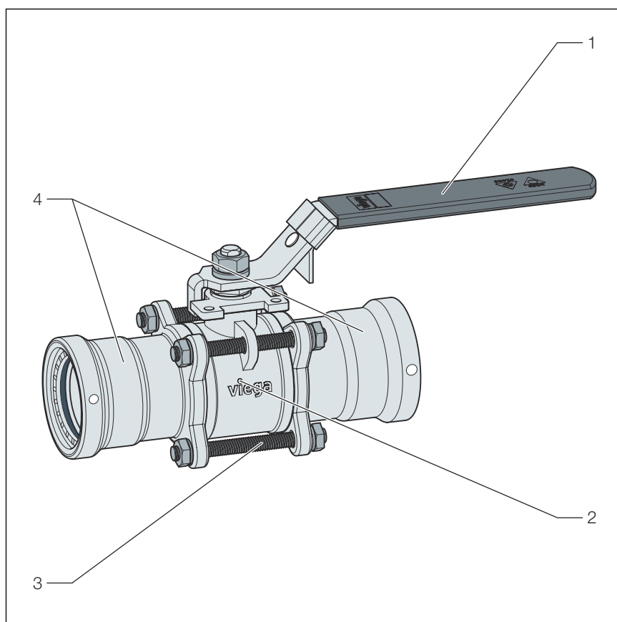
Abb. 2: dreiteiliger Kugelhahn
