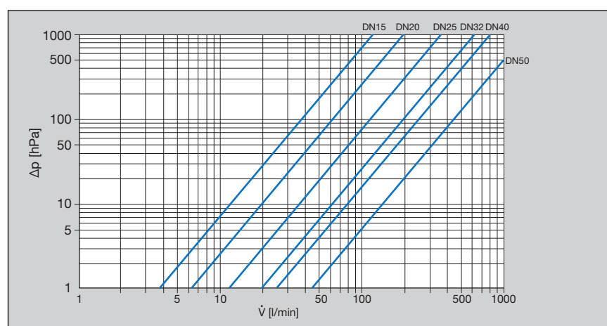
Abb. 3: Leistungsdiagramm Schrägsitzventile Press-/Gewindeanschluss
