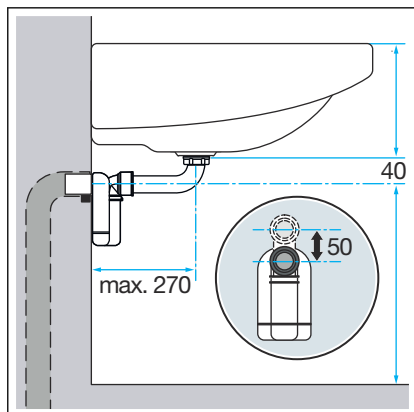
Obr. 2: Montážne rozmery
