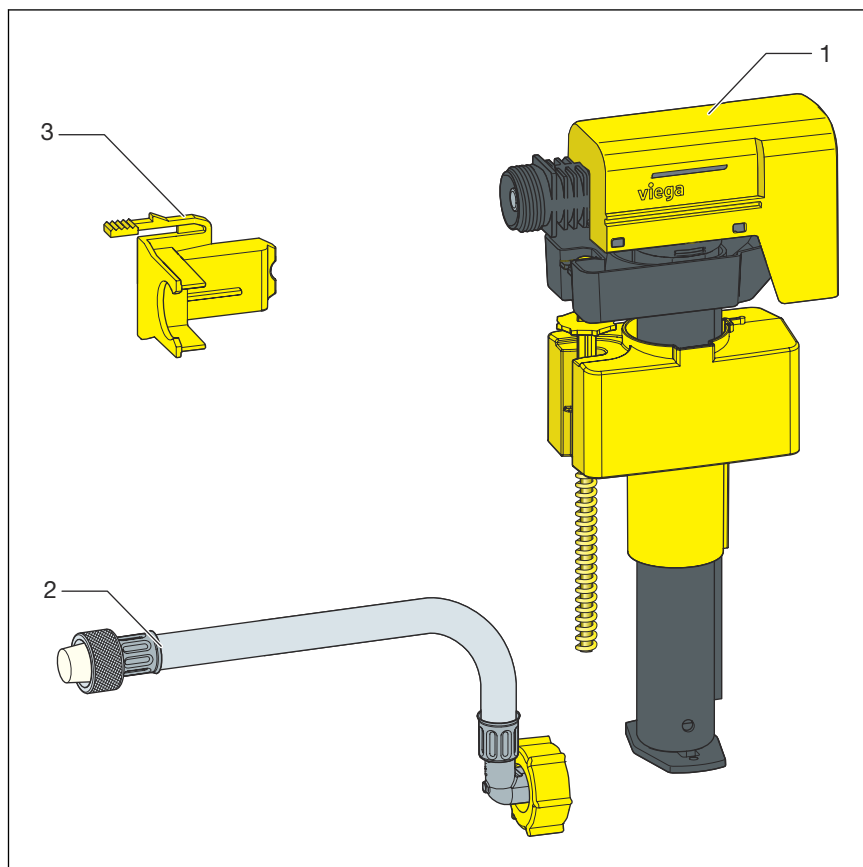
Fig. 1: Conjunto de válvula de enchimento
