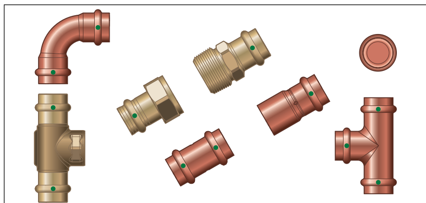
Fig. 1: Seleção de produtos Profipress
