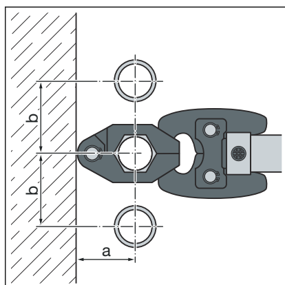
Prensar entre o tubo e a parede
