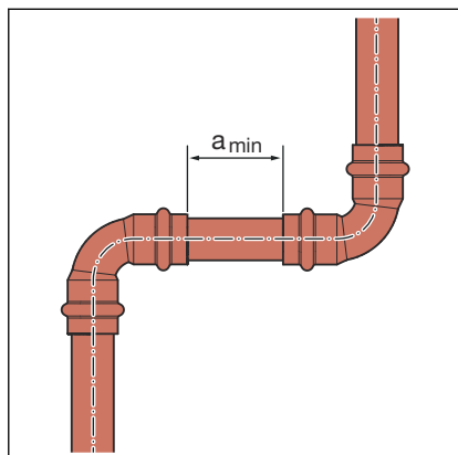
Distância mínima nos mordentes de prensar d 12–54
