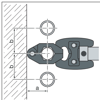
Izvođenje press spojeva između cijevi i zida
