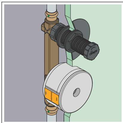
Slika 4: 2235.90 prednji pričvrсни set
