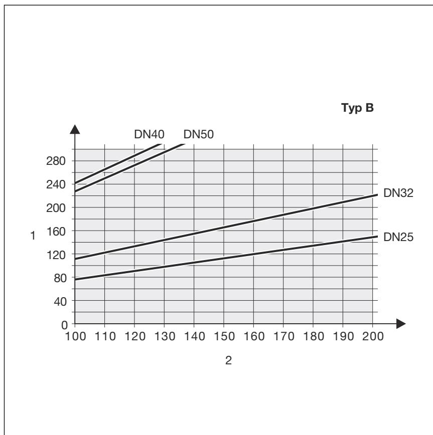
5. ábra: Irányadó értékek megfűróidomhoz és főelzáróhoz, \zeta=10 alaki ellenállástényezőhöz
