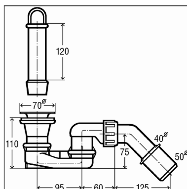
Abb. 2: Maßzeichnung
