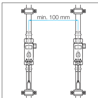
Abb. 7: Abstand zwischen zwei AquaVip-Zirkulationsregulierungsventilen
