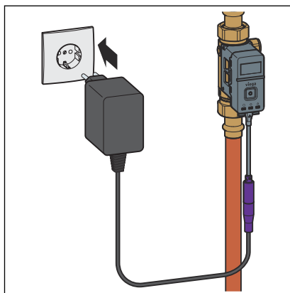
Abb. 4: Netzteil und AquaVip-Zirkulationsregulierventil elektronisch im eingebauten Zustand
