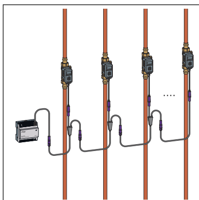
Abb. 6: AquaVip-Netzteil und x AquaVip-Zirkulationsregulierventile, Spannungsversorgung mit AquaVip-Y-Kabel
