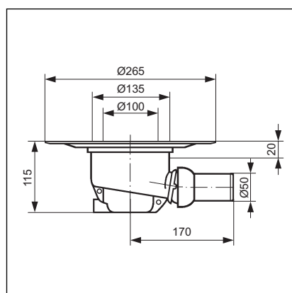
Bild 7: Ritning modell 4921.3
