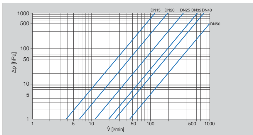
Abb. 3: Leistungsdigramm Schrägsitzventile Press-/Gewindeanschluss
