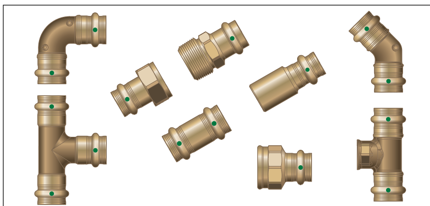
Rys. 1: Złączki zaprasowywane Sanpress
