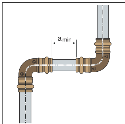
Minimalna odległość przy szczękach zaciskowych d15–54
