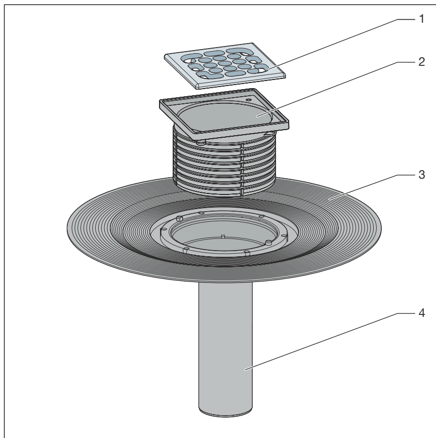
Fig. 1: Componenti scarico per terrazze e balconi modello 4944.2
