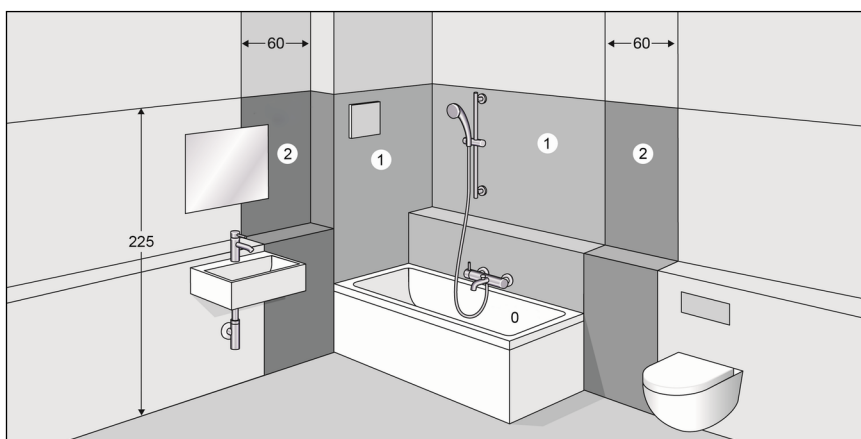
Abb. 18: Schutzbereiche nach VDE 0100 Teil 701
