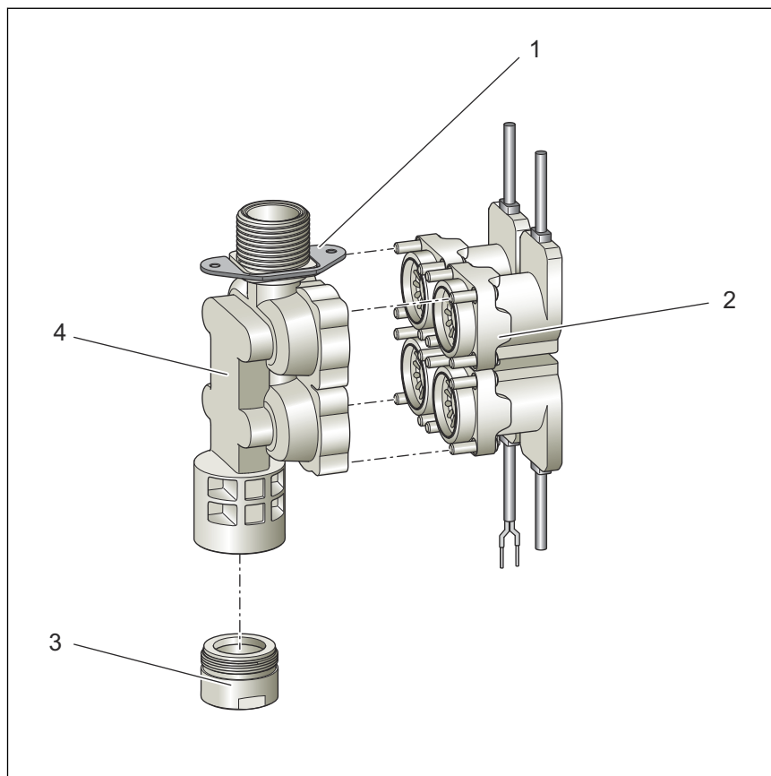
Abb. 3: Übersicht Magnetventil
