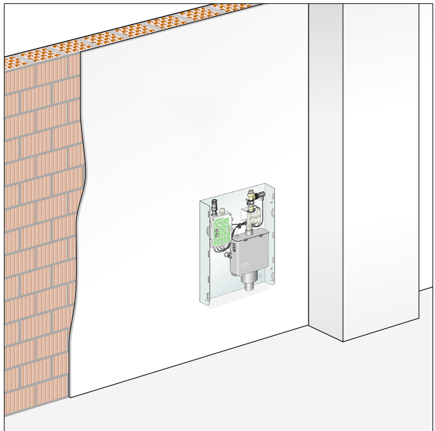
Abb. 11: Einbauschema Aufputz
