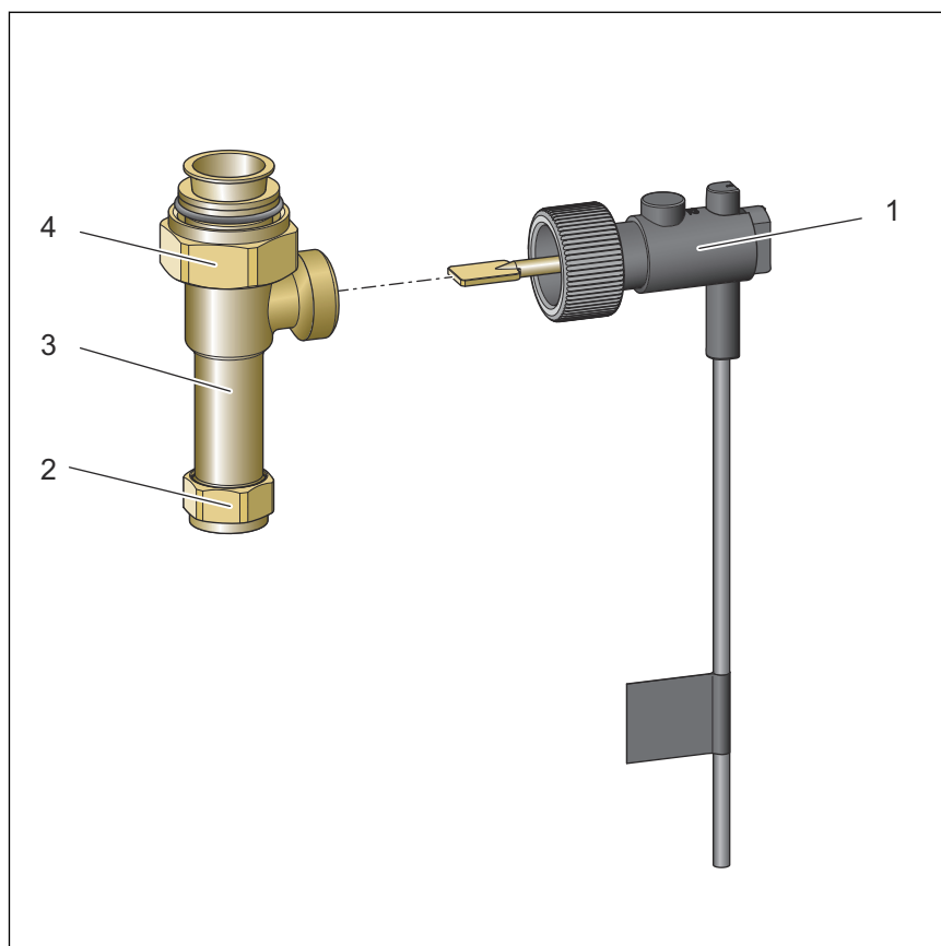
Abb. 4: Übersicht Strömungsschalter
