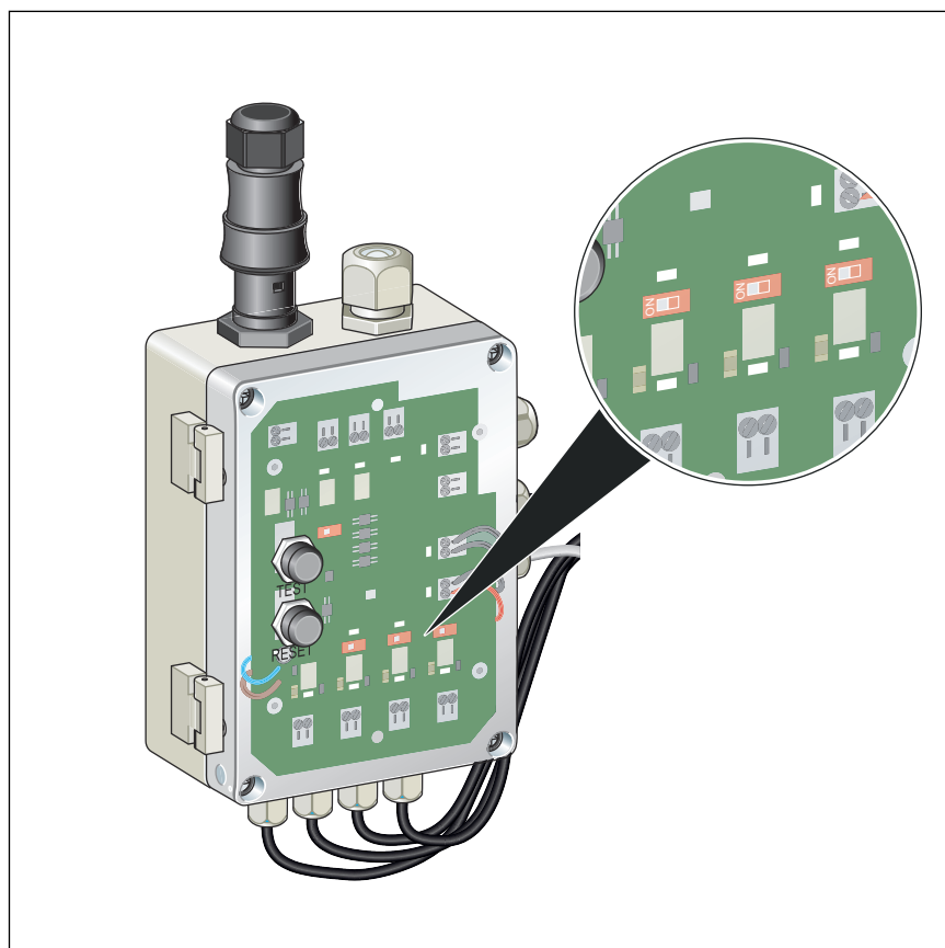
Abb. 20: Steuerung Schalterstellung ON
