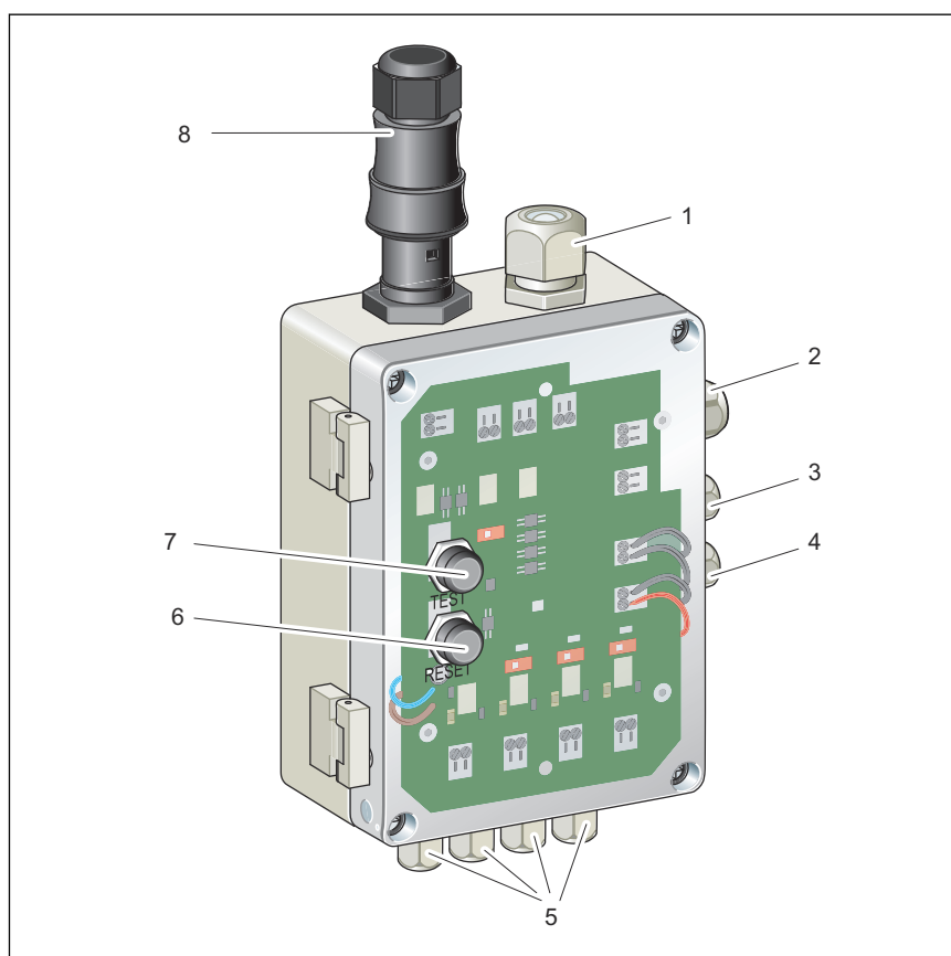
Abb. 17: Übersicht Steuerung
