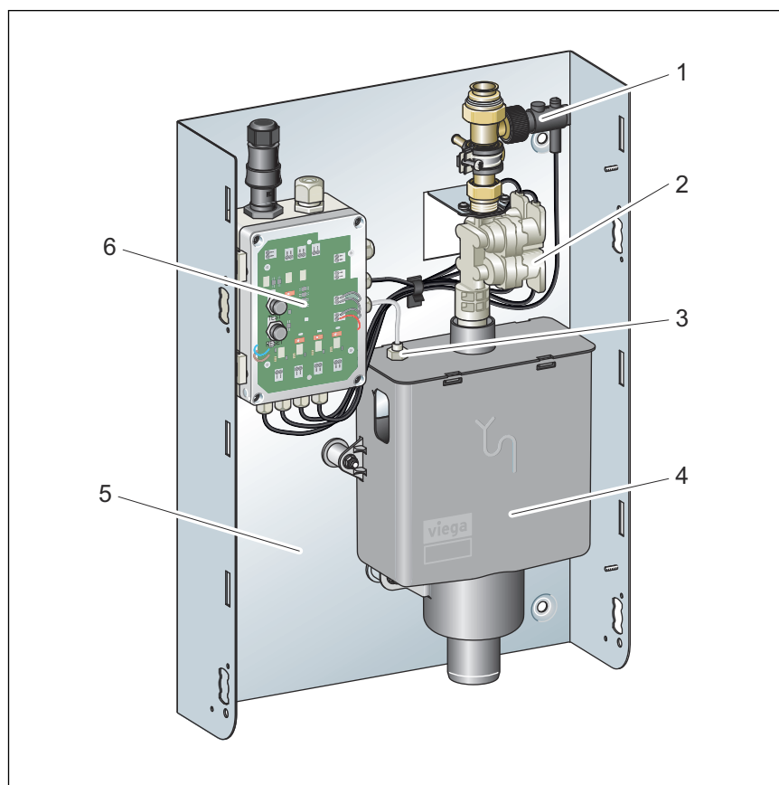
Abb. 1: Übersicht Spülventil
