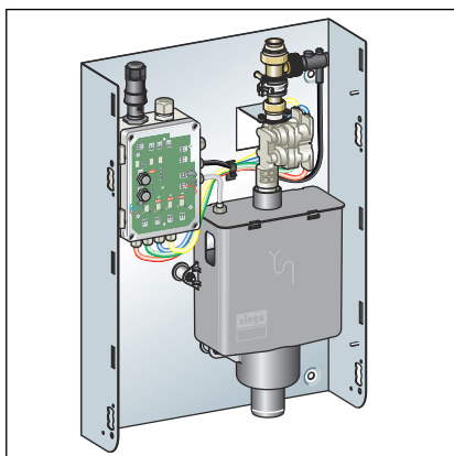
Abb. 21: Kabelverbindungen
