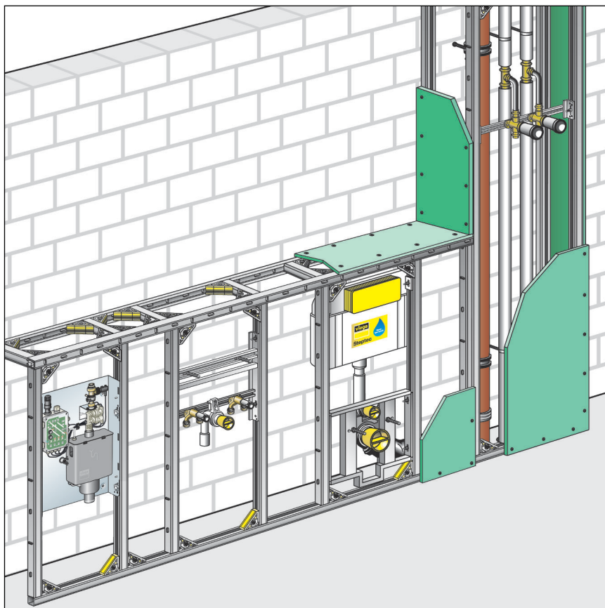
Abb. 7: Einbauschema Viega Steptec
