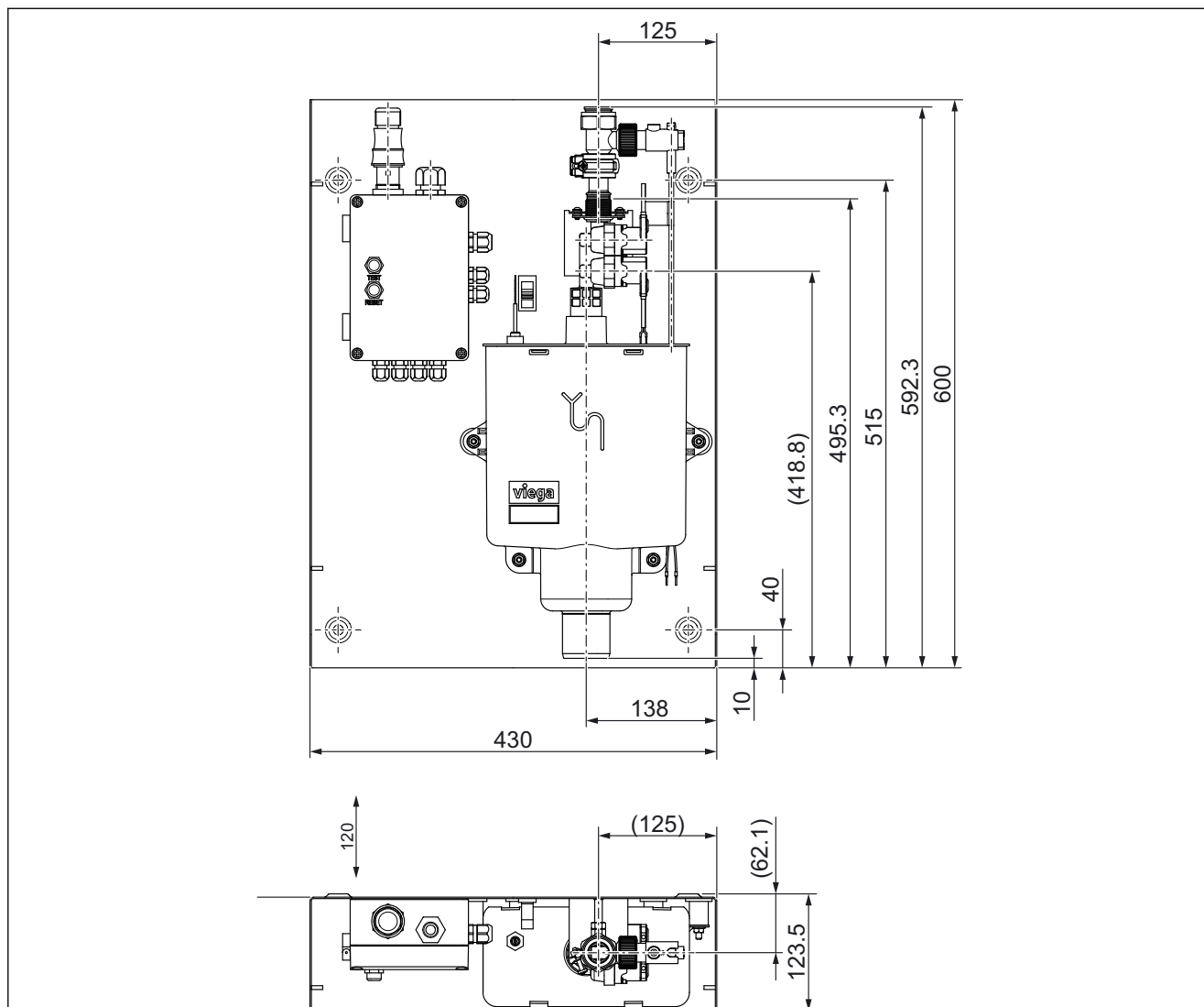
Abb. 13: Abmessungen Spülventil
