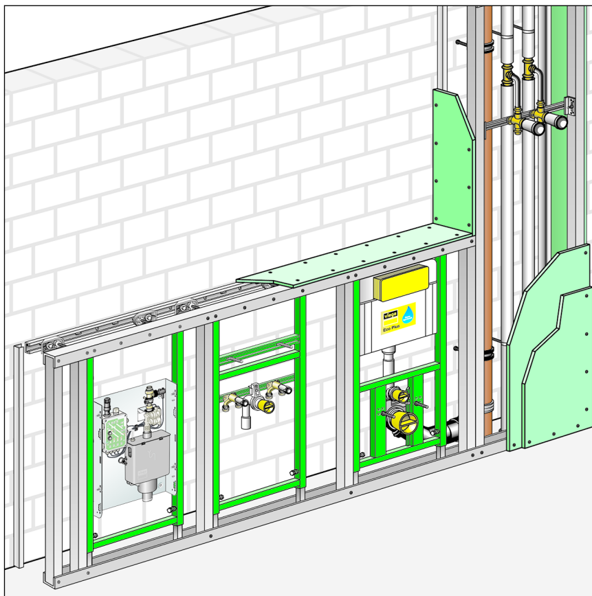
Abb. 9: Einbauschema Viega Eco Plus
