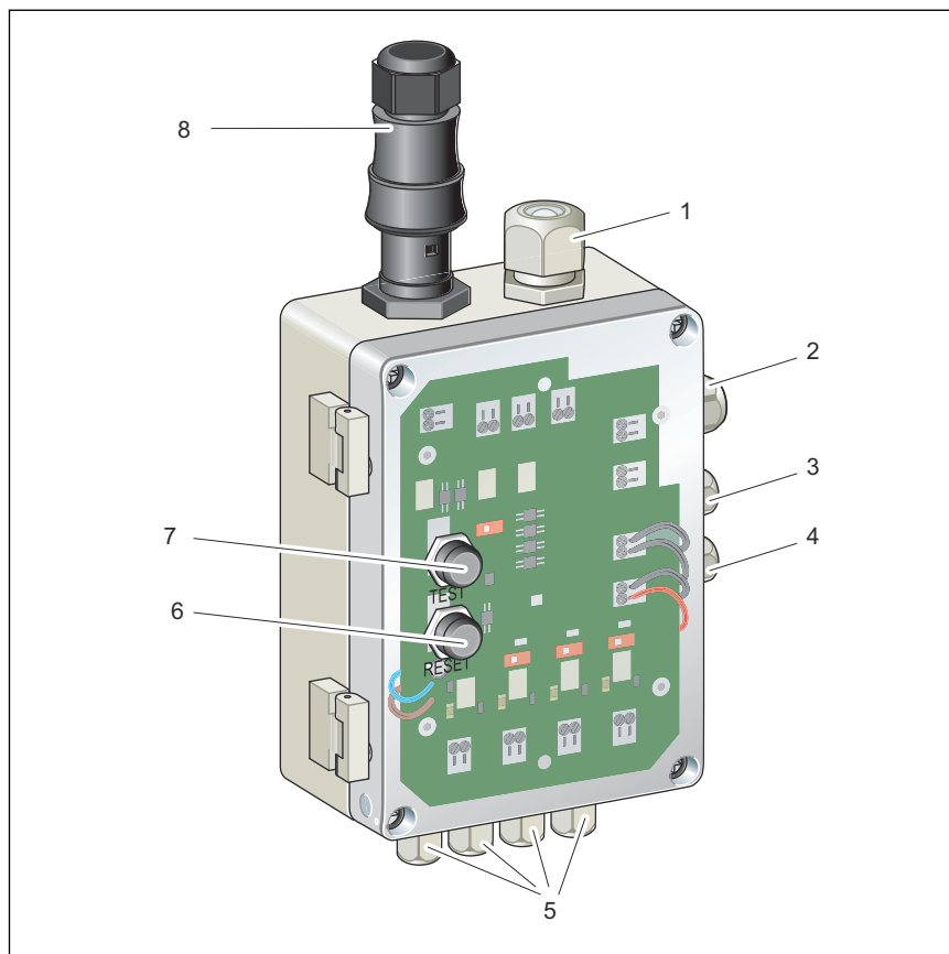
Abb. 2: Übersicht Steuerung
