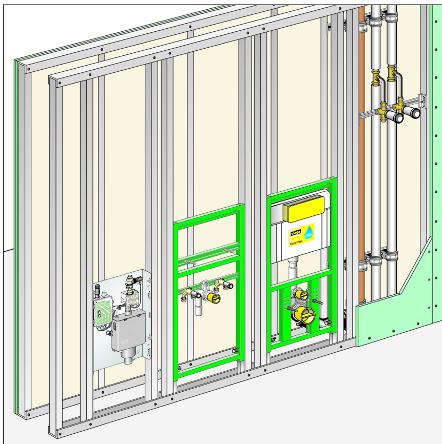
Abb. 12: Einbauschema Trockenbau
