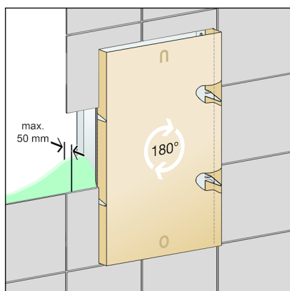
Abb. 19: Schutzkarton
