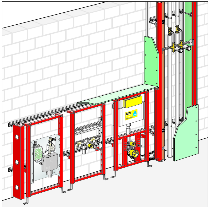
Abb. 8: Einbauschema Viegaswift
