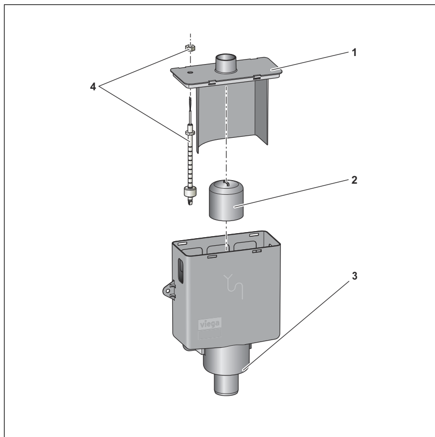
Abb. 5: Übersicht Siphon
