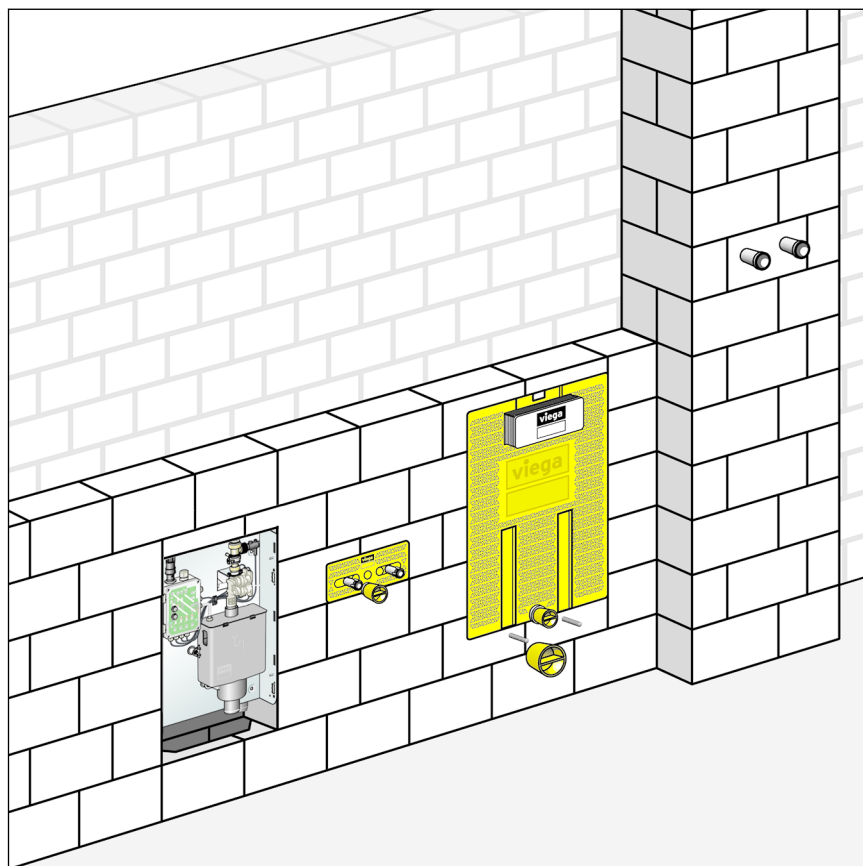
Abb. 10: Einbauschema Unterputz
