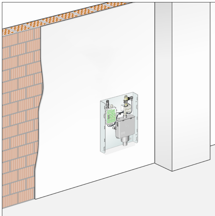
Abb. 11: Einbauschema Aufputz
