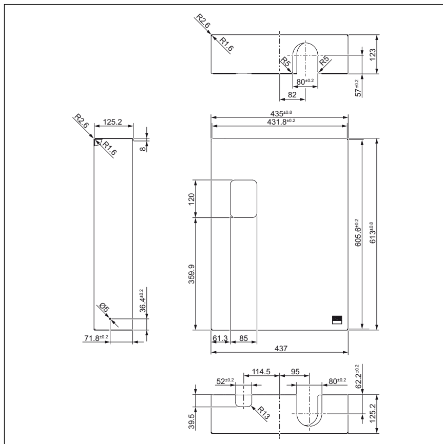
Abb. 15: Abmessungen Aufputzabdeckung
