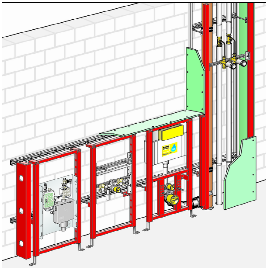
Abb. 8: Einbauschema Viegaswift
