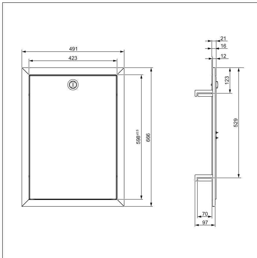
Abb. 14: Abmessungen Unterputzabdeckung
