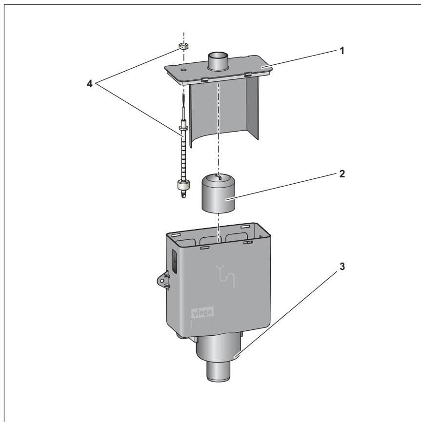
Abb. 5: Übersicht Siphon
