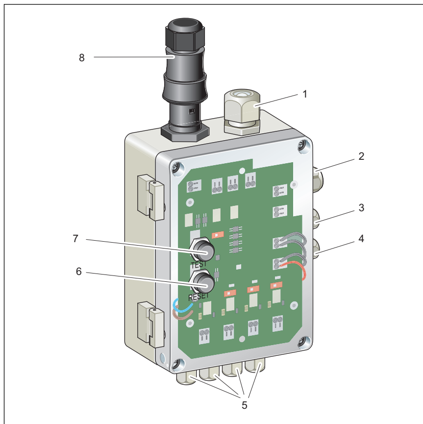
Abb. 17: Übersicht Steuerung
