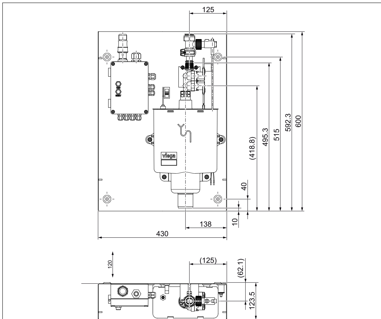
Abb. 13: Abmessungen Spülventil
