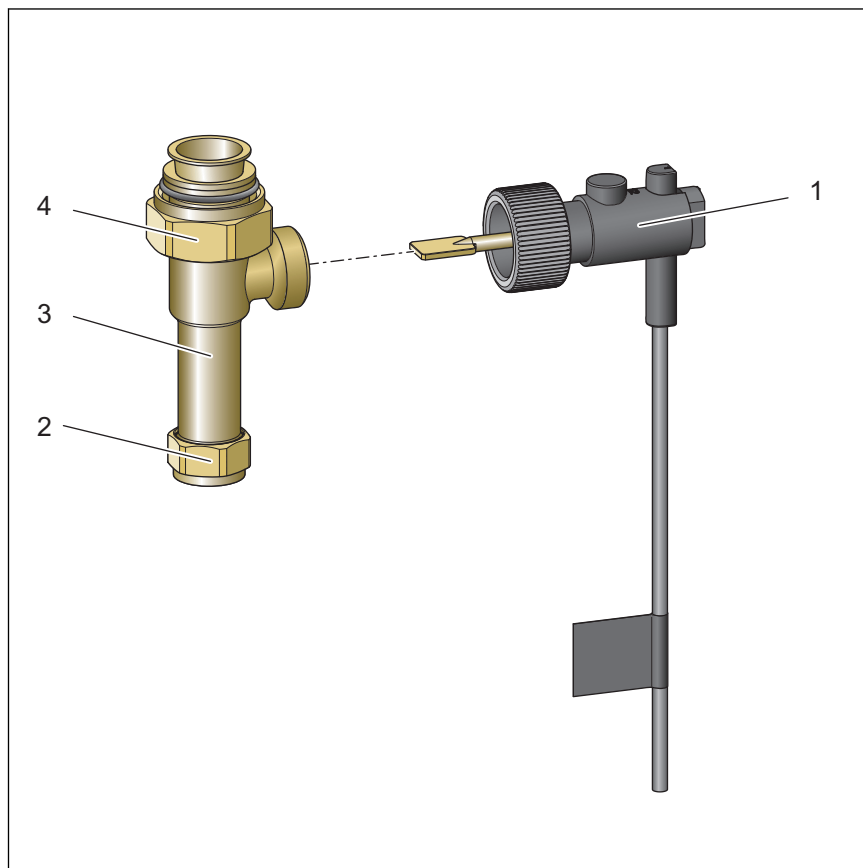
Abb. 4: Übersicht Strömungsschalter
