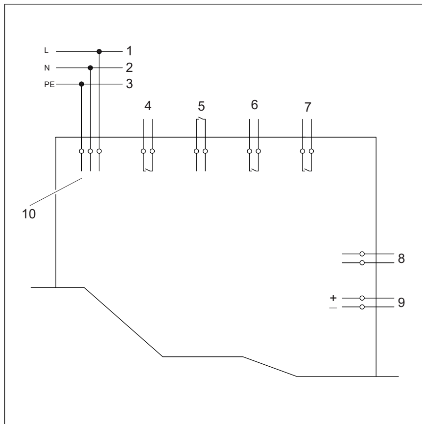
Abb. 6: Anschlussplan
