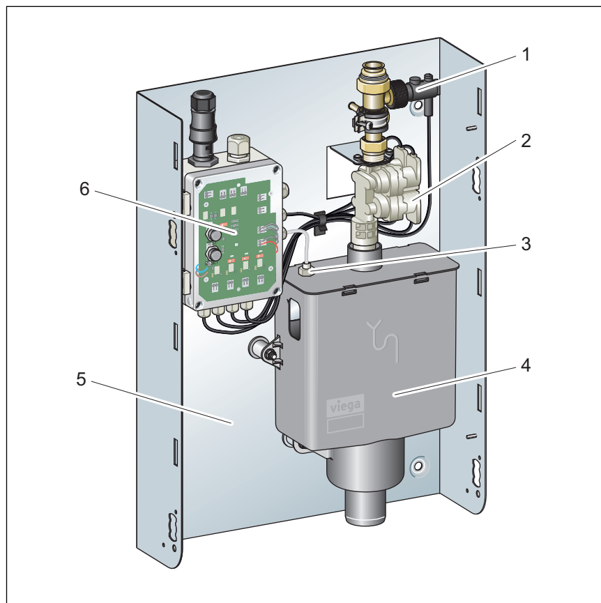
Abb. 1: Übersicht Spülventil
