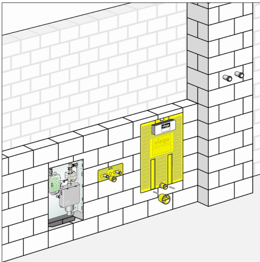
Abb. 10: Einbauschema Unterputz
