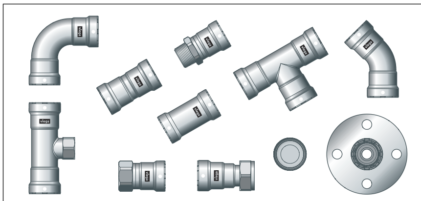
Obr. 2: lisovacie spojky Megapress S
