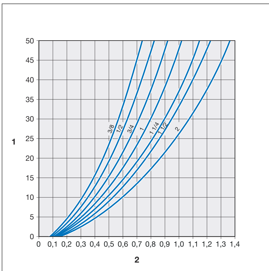
Obr. 7: rameno ohybu tvar U pre Megapress S 3/8 až 2 cölý
