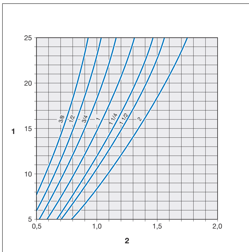
Obr. 5: rameno ohybu tvar Z a T pre Megapress S 3/8 až 2 cölý
