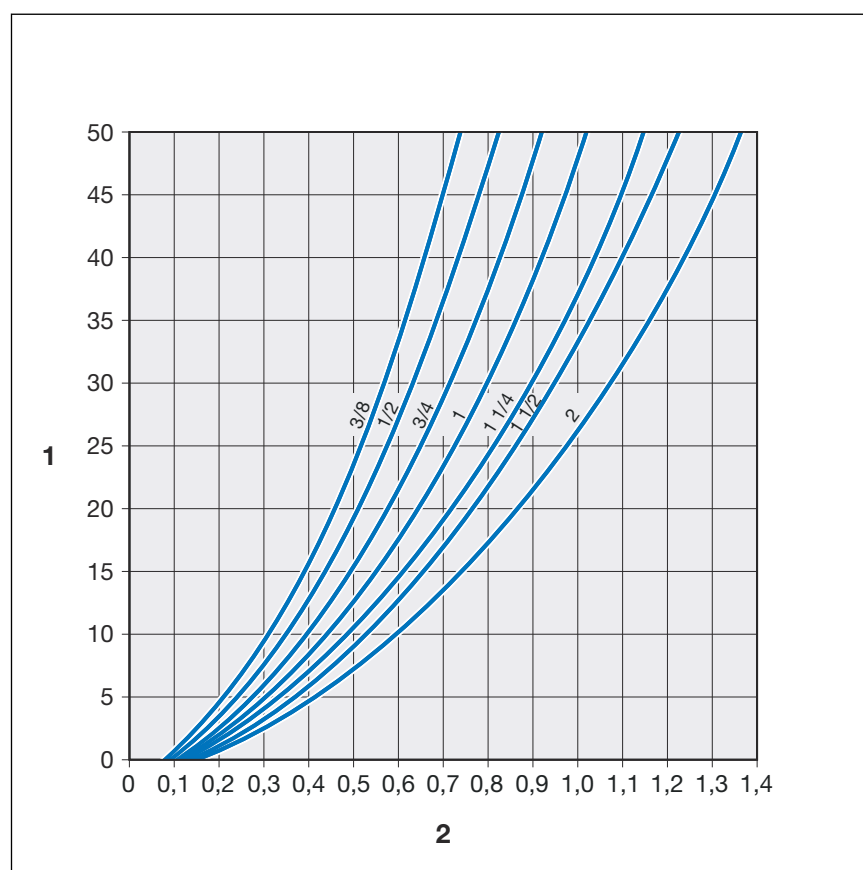
Fig. 7: Curvatura em forma de U para Megapress S ½ até 2 polegadas
