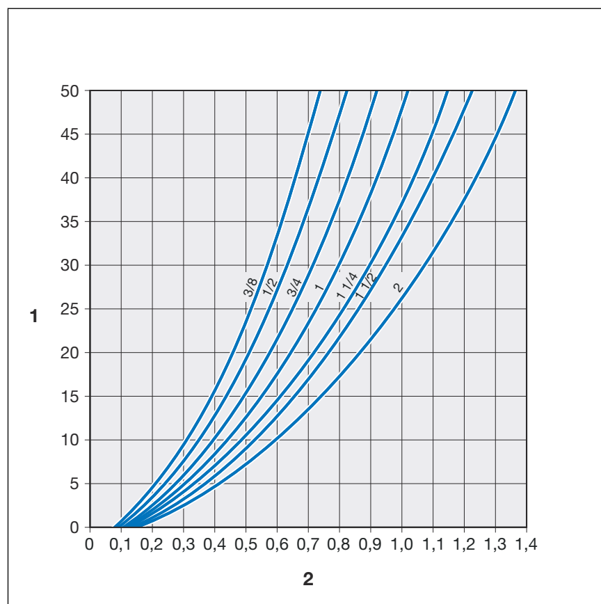
Rys. 7: Ramię elastyczne w kształcie U do Megapress S % do 2"
