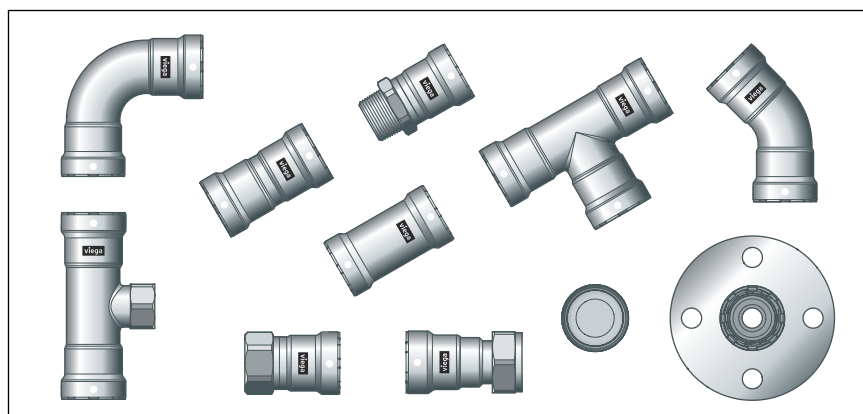
Rys. 2: Złączki zaprasowywane Megapress S
