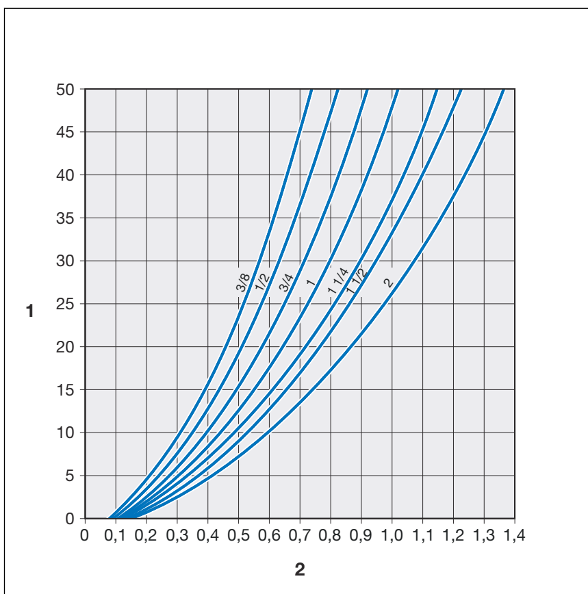
7. ábra: Hajlítás, U-alak, Megapress S 3/8-2 col között
