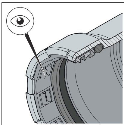
15. ábra: Vágógyűrű
