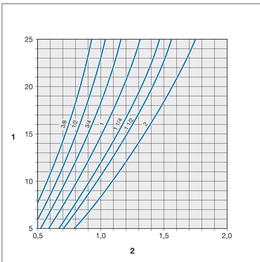
5. ábra: Hajlítás, Z- és T-alak, Megapress S ¾-2 col között
