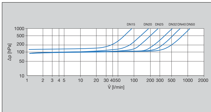
Slika 1: Dijagram učinka, pad tlaka, KRV, press/navojni priključak
