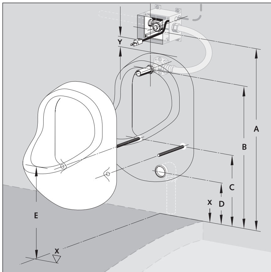
Slika 2: Dimenzije instalacije
