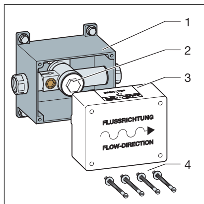
Slika 1: Komponente
