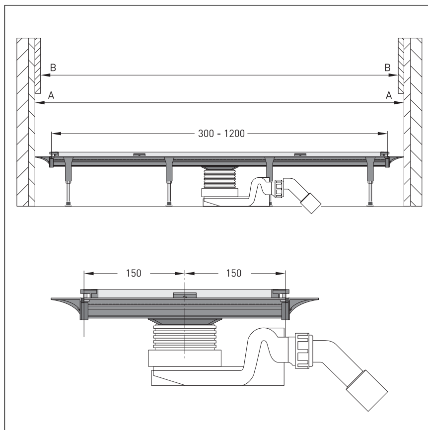
Slika 18: Dimenzije niše
