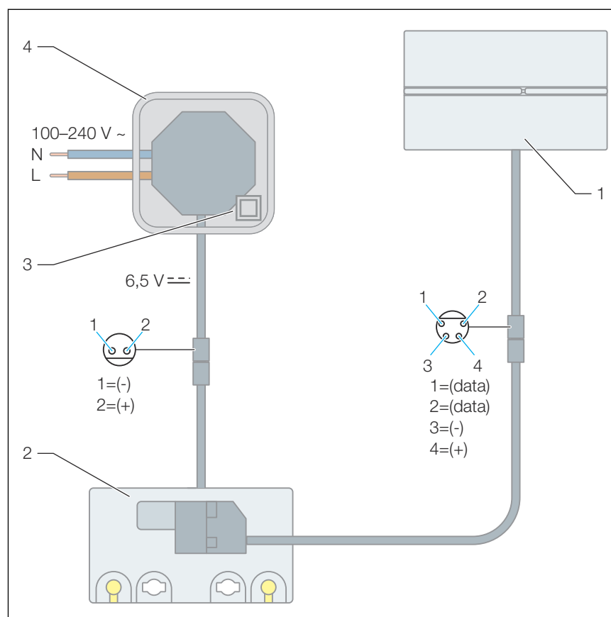
Fig. 2: Schema di collegamento, alimentatore di rete, piastrina di comando per WC per Prevista
