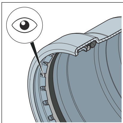
Rys. 11: Pierścień nacinający
