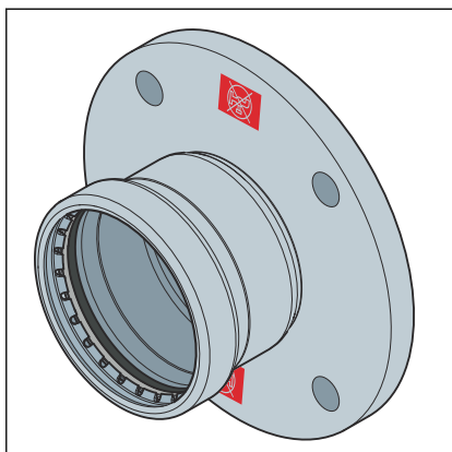
Rys. 13: Kolnierz stały 1159.1XL
