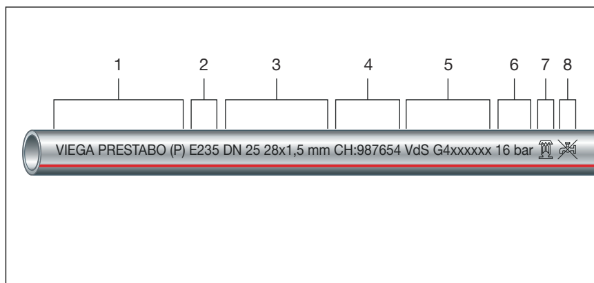
Fig. 7: Tubo zincato sendzimir internamente e esternamente
