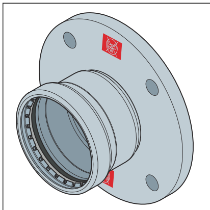
Abb. 13: Festflansch 1159.1XL
