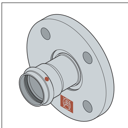
Afb. 11: Vaste flens
