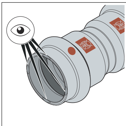
Afb. 9: Inkepingen Temponox
