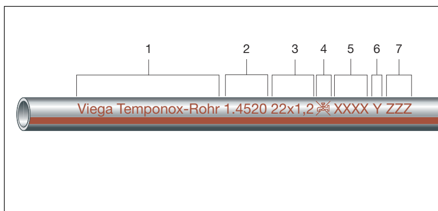
Abb. 6: Temponox-Rohr 1.4520
