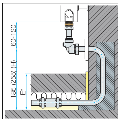
Obr. 9: Montážne rozmery
