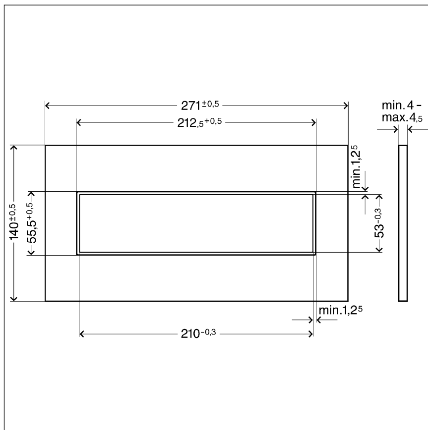
2. ábra: Méretraajz, 8332.3
