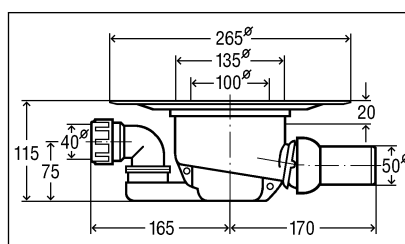
Bild 7: Ritning modell 4921.65
