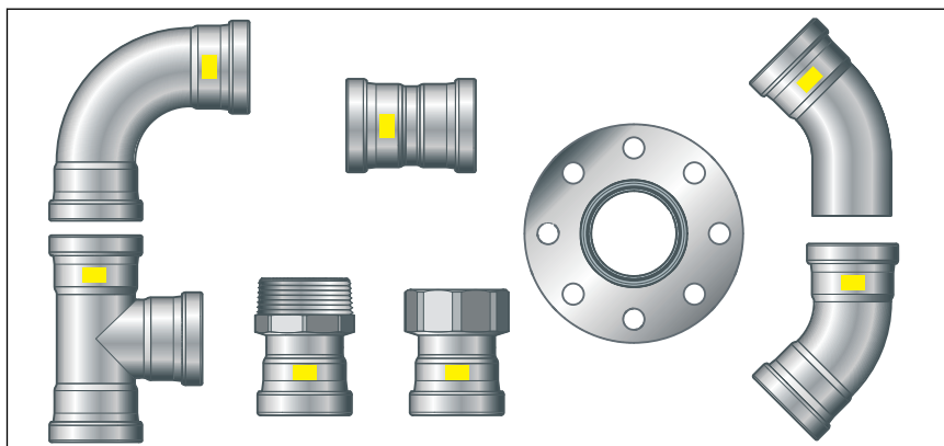
Obr. 1: lisovacie spojky Sanpress Inox G XL
