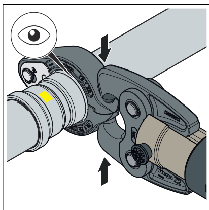
Obr. 5: Otvorenie čeluste s kĺbovým ťahom Sanpress Inox G XL
