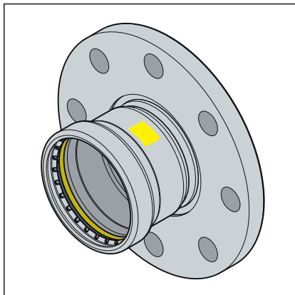
Obr. 6: Pevná prírub
