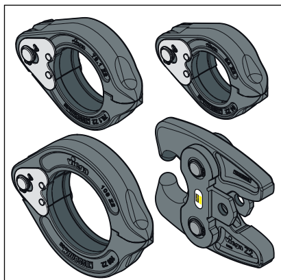
Obr. 4: lisovacie prstence a čelúšť s kĺbovým ťahom
