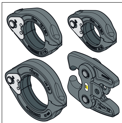
Fig. 4: Anillos de prensar y mordaza articulada
