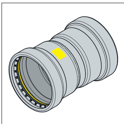
Obr. 2: Lisovací spojky
