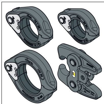
Obr. 4: Lisovací prstence a tahná kloubová čelist
